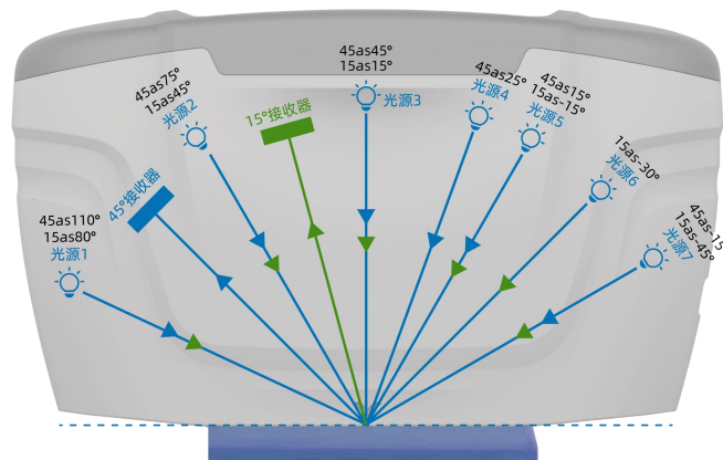
测量原理图
